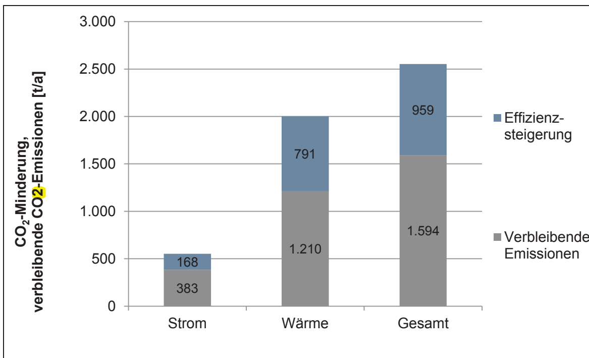
Abbildung 26: Theoretische CO 2 -Minderungspotenziale und verbleibende Emissionen
